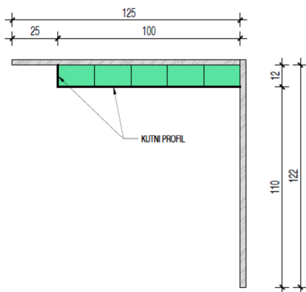
TLOCRT
