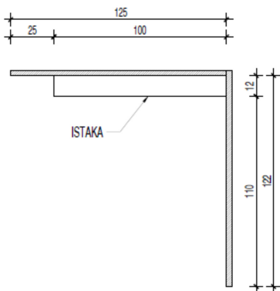
TLOCRT
